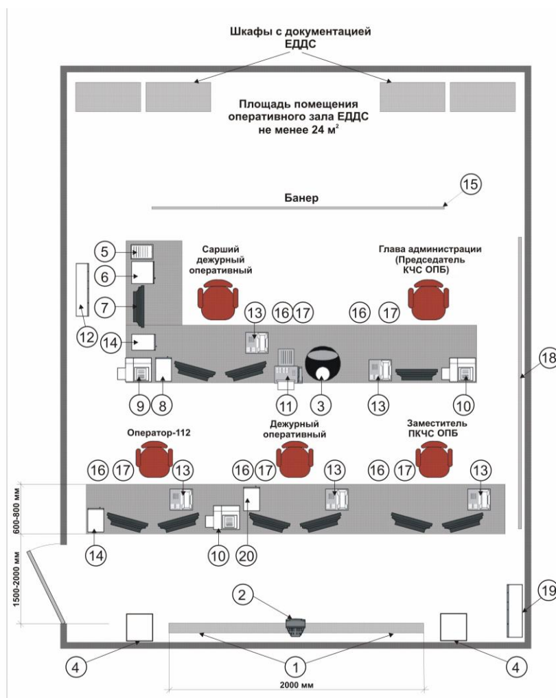
Рисунок А.1 – Примерная схема размещения рабочих мест и оборудования ЕДДС
